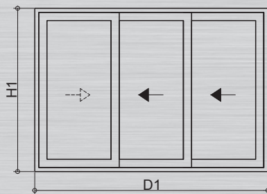
ANSICHT 3-TEILIGE SCHIEBETÜR
